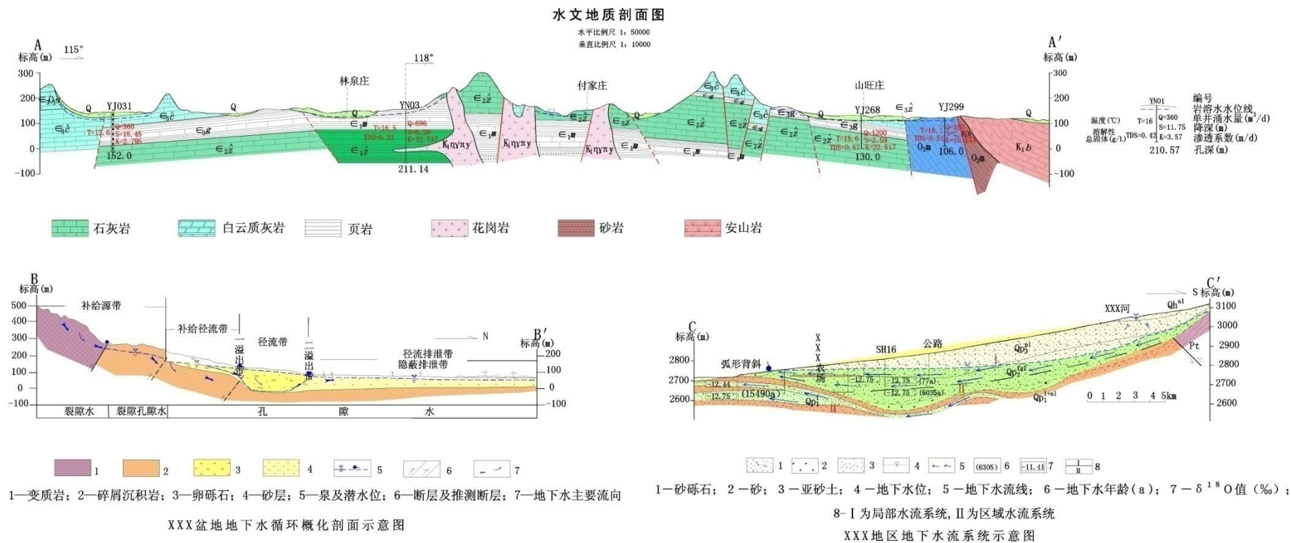
图A.4 水文地质剖面图示例
