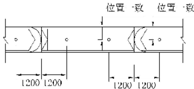
图 10.1.4 注浆管安装位置示意图
